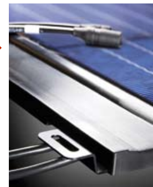
Gros plan technique sur la connectique, les fixations intégrées et le cadre de KoraSun® : facilité de mise en œuvre pour une longévité élevée.
